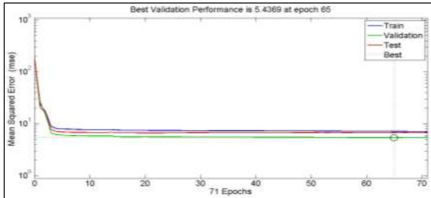
الشكل (6) : مسار تدريب الشبكة العصبية الاصطناعية لنموذج ESDP باستخدام خوارزمية التدريب (Levenberg Marqwardt LM)
